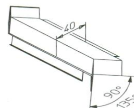
vnitřní roh
