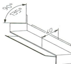
vnější roh
